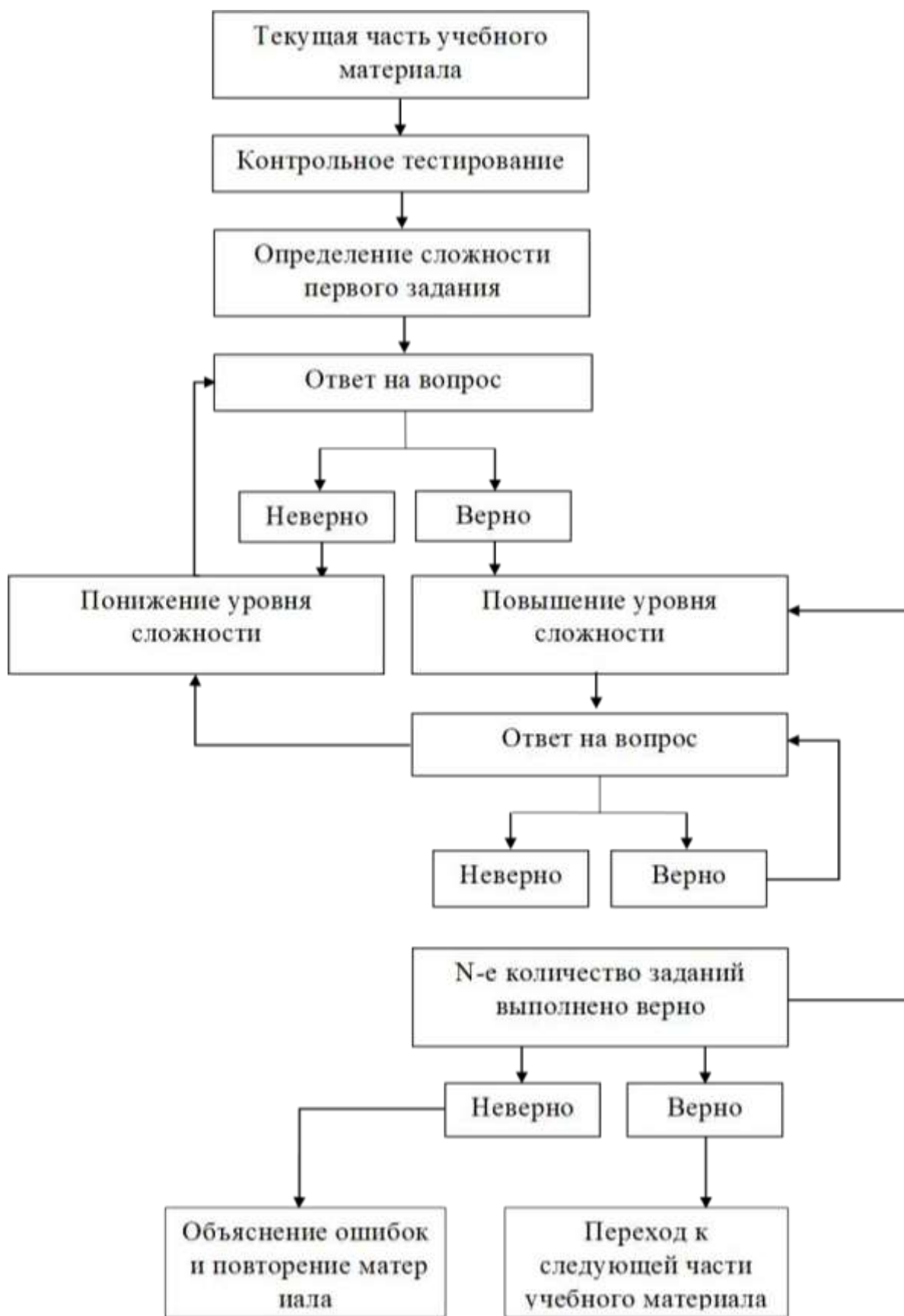
Схема 3 — Алгоритм адаптивной программы
