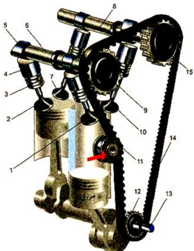
Рис. 2.9 – ГРМ с двумя распределительными валами:
