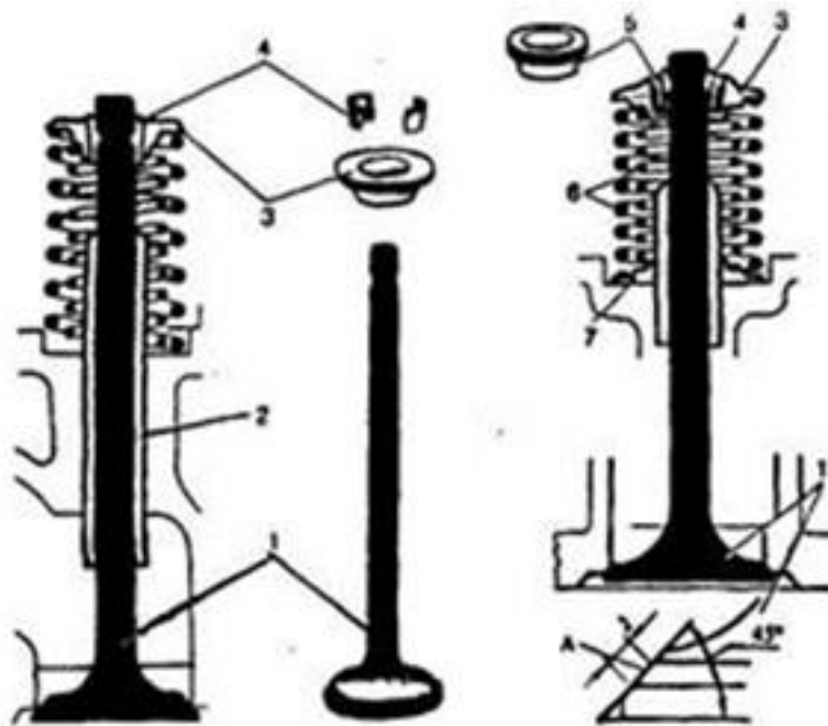
Рис. 2.12 – Клапанный механизм:
