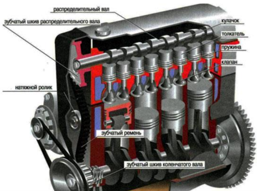
Рис. 2.2 – Устройство верхнеклапанной системы ГРМ четырехтактных ДВС
