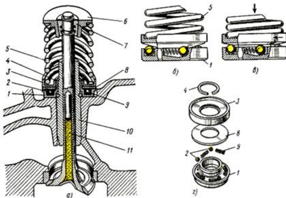
Рис. 2.13 – Выпускной клапан:
