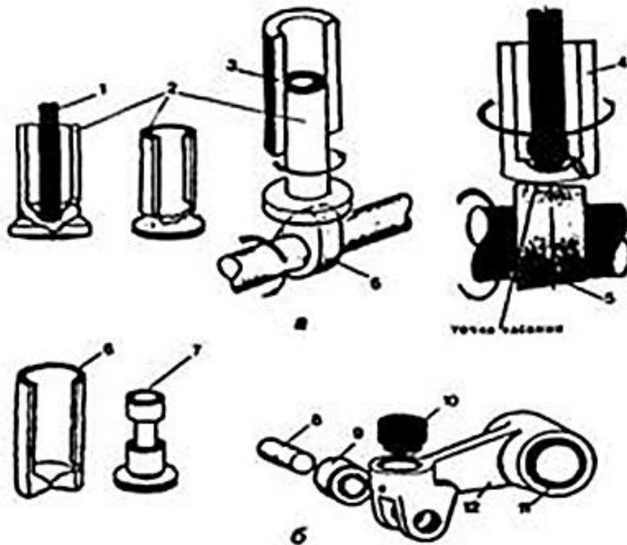
Рис. 2.10 – Толкатели:
