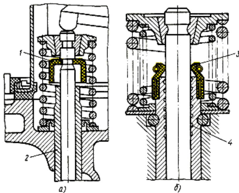
Рис. 2.14 – Уплотнения клапанов:
