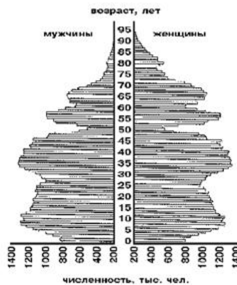
Рисунок 1 Половозрастная пирамида [11]
