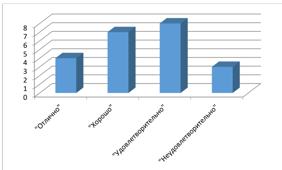
Рис 1. Результаты тестирования
