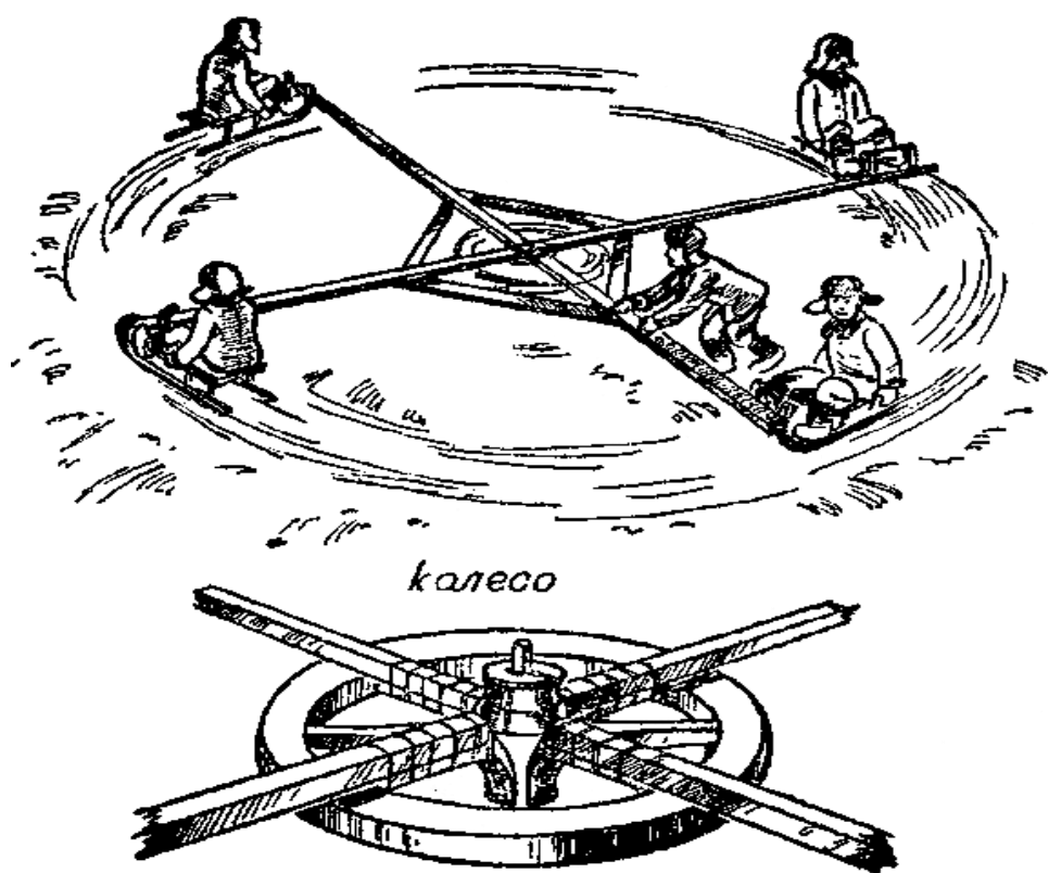
Рис. 9. Устройство деревенской карусели или «кружало»
