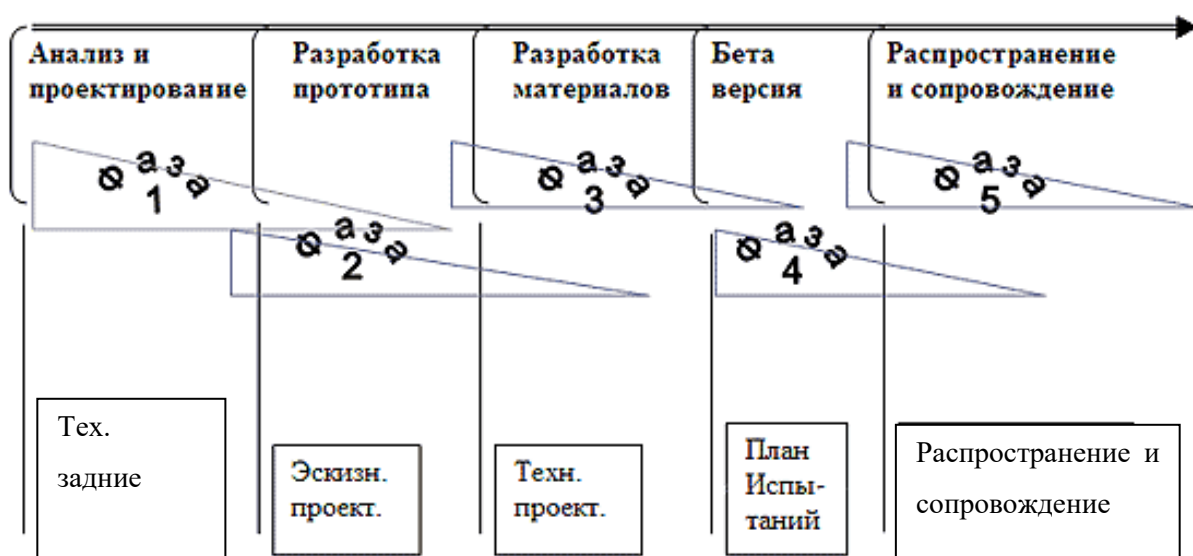
Рисунок 8. Модель Эшера
