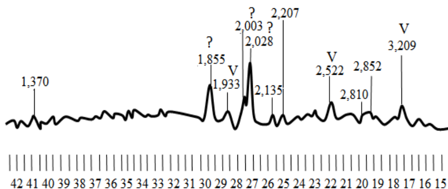
V - CaAl_2Si_{1,5} (1,933; 2,522; 3,209)
