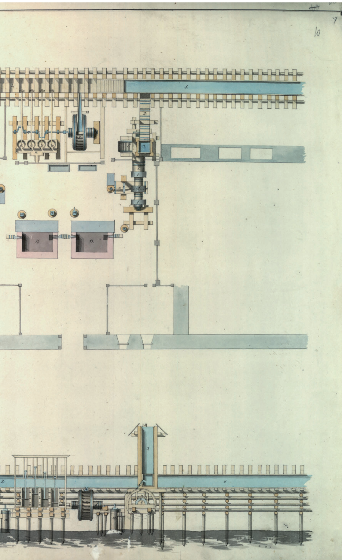
План и фасады стальной фабрики Изъяснение
