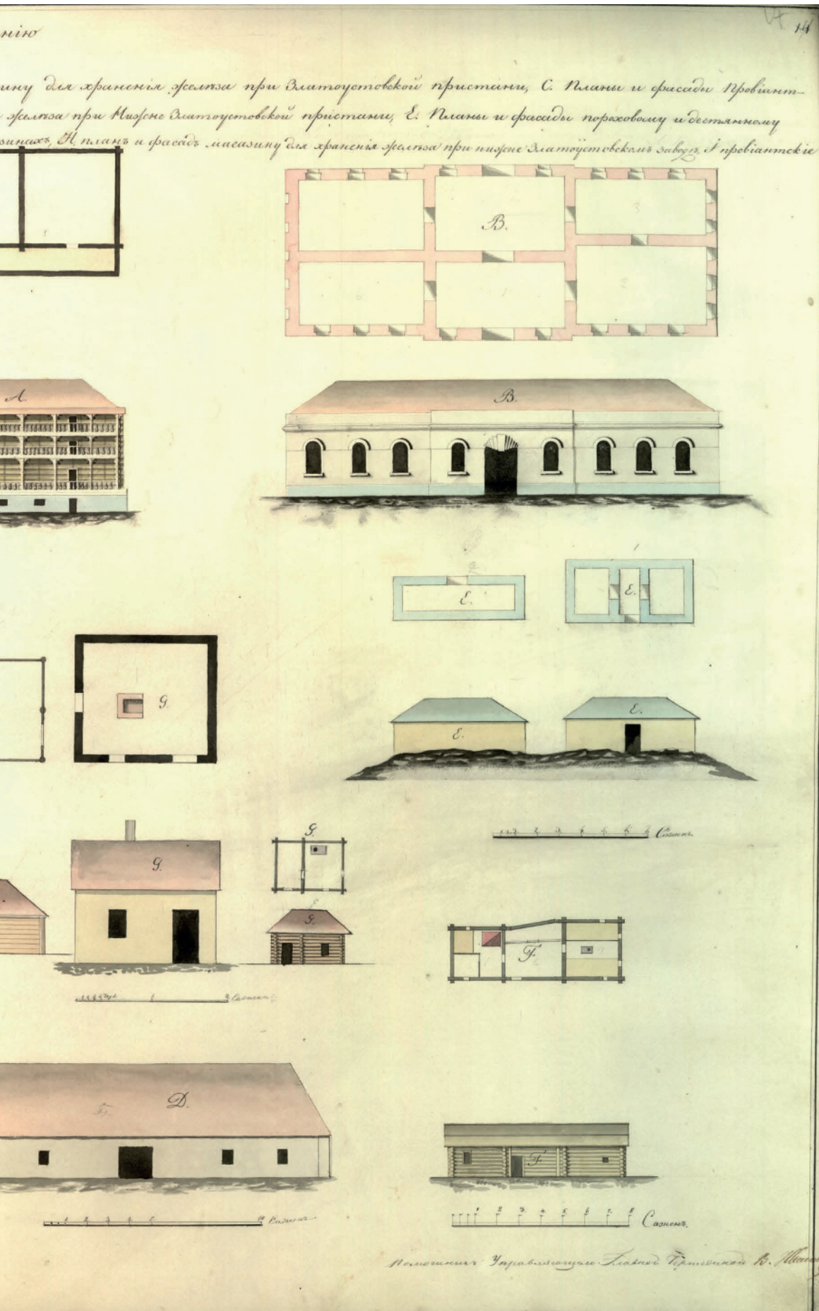
Планы и фасады казенному строению Изъяснение
