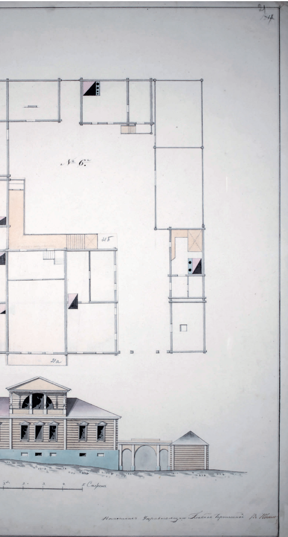
Планы и фасады казенным домам для жительства гг. чиновников
