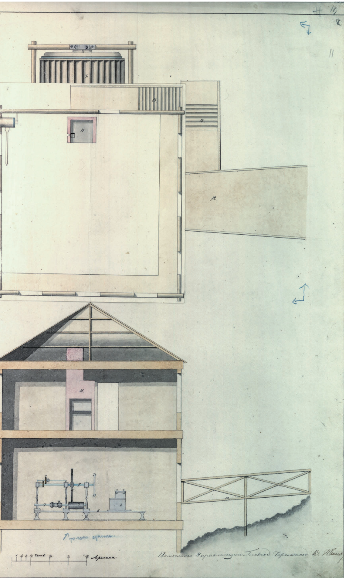
План, фасад и профиль токарной фабрики Изъяснение
