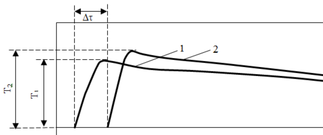
Рис. 2 Кривые температуры горения азидных СВС-систем: 1 - показания первой термопары; 2 - показания второй термопары; T_1 - температура горения шихты регистрируемая 1-й термопарой, °С; T_2 - температура горения шихты регистрируемая 2-й термопарой, °С; \Delta\tau - время прохождения фронта горения между термопарами, сек
