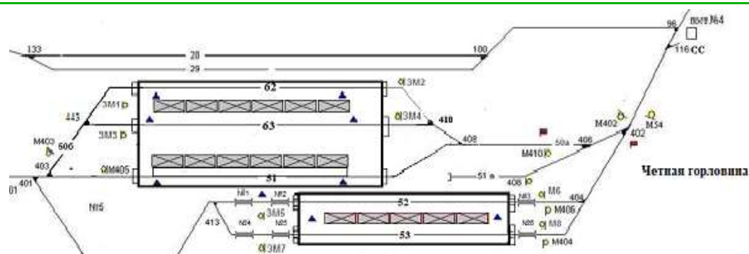
Рис.3 Новая эстакада на 51пути
