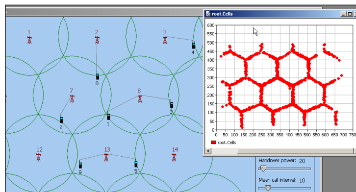
Рис.4.4. AnyLogus - модель сотовой телекоммуникационной системы.
