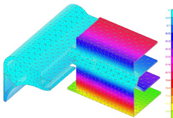
Рис. 1.9. Отображение результатов расчета температурных полей.
