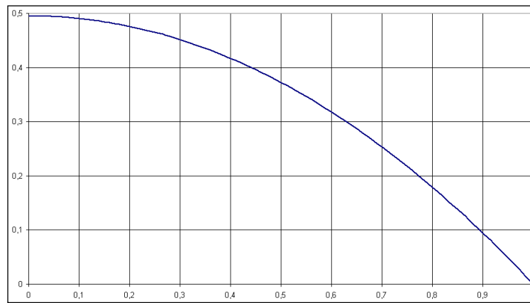
Рис.2.30. Результат расчета профиля скорости ламинарного течения жидкости.
