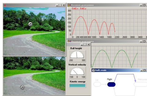
Рис. 3.17. Представление результатов моделирования движения упругого мяча.
