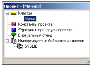
Рис.1.8. Проект MVS.
