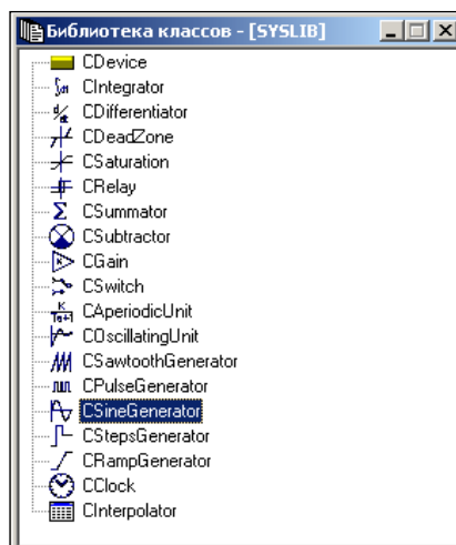
Рис. 1.18. Библиотека классов.
