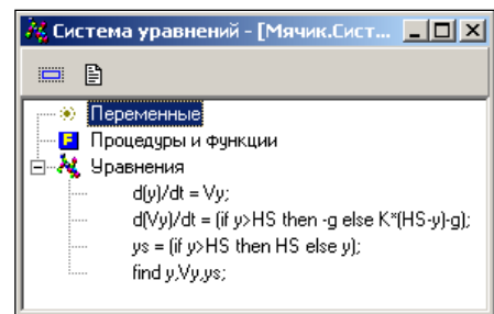
Рис. 1.11. Система уравнений.
