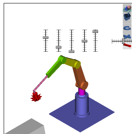
Рис. 1.7. Модель манипулятора.
