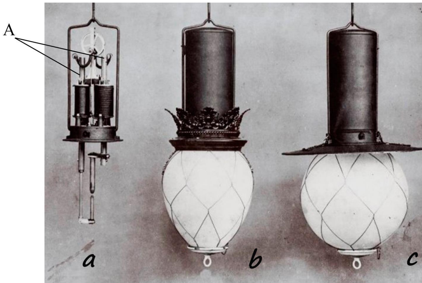
Рисунок 11. Конструкция и внешний вид дуговой лампы с использованием электрода. [Мокрецова А.П.,2022]
