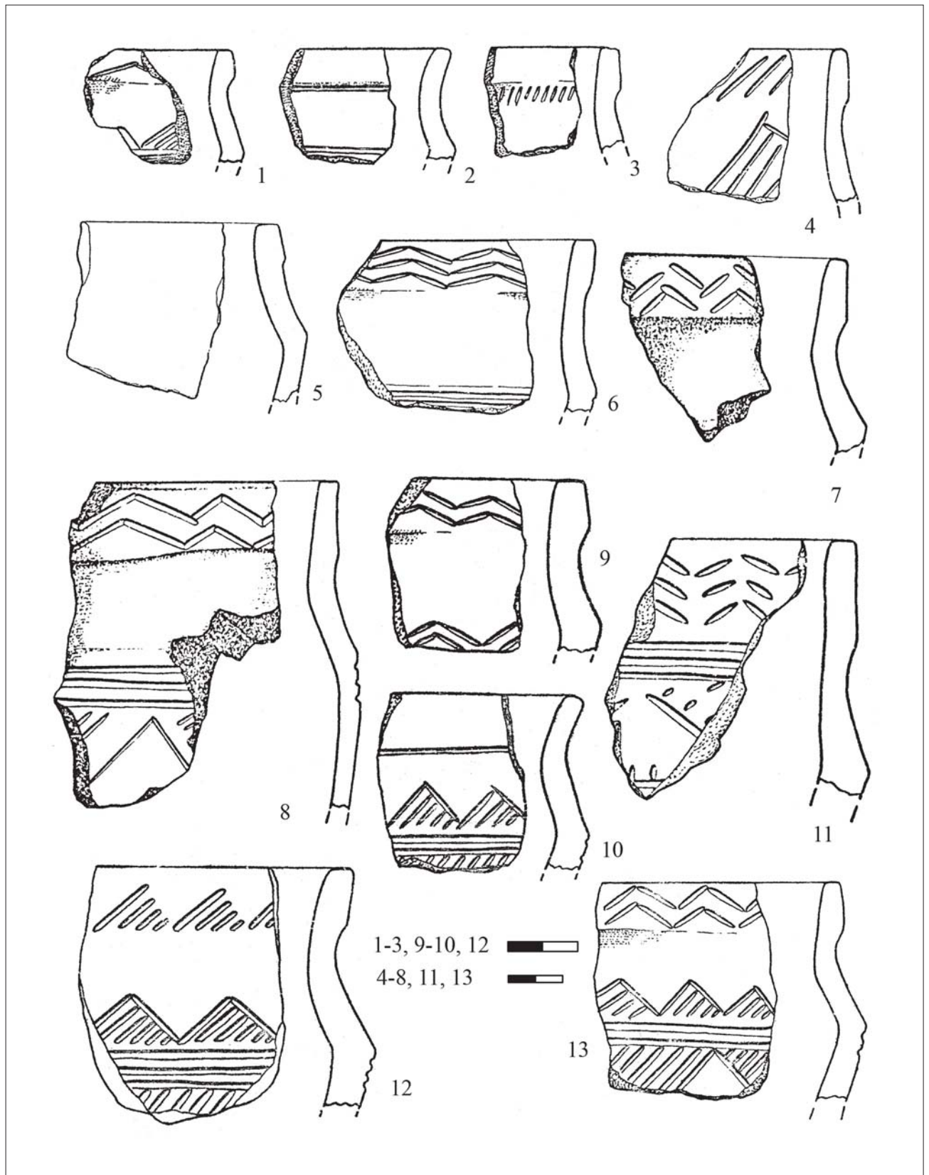
Рис. 35. Керамика памятников петровского типа
