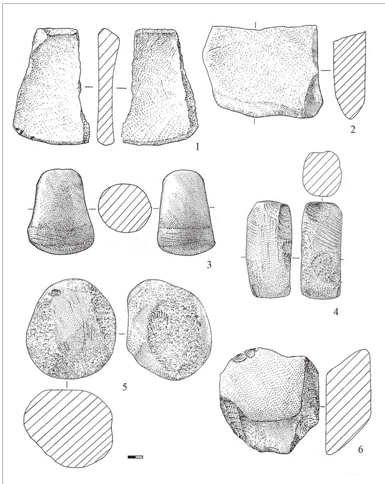
Рис. 16. Памятники синташтинского типа. Каменные орудия металлургии и металлообработки. Укрепленное поселение Синташта I
