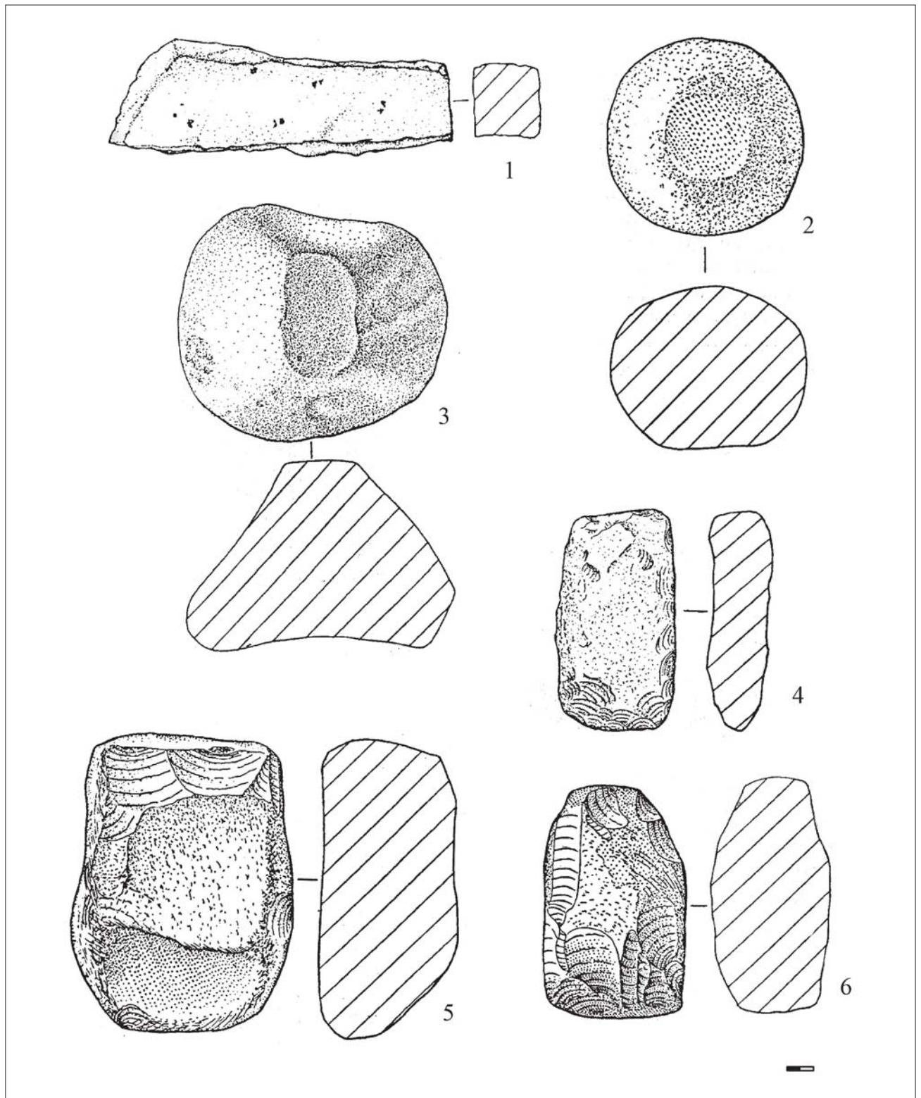
Рис. 17. Памятники синташтинского типа. Каменные орудия металлургии и металлообработки. Укрепленное поселение Аркаим. Каменные орудия 1 – терочник; 2 – пест; 3 – подставка-наковальня; 4 – молоток; 5–6 – молот. По: (Зайков, Зданович, 2000)
