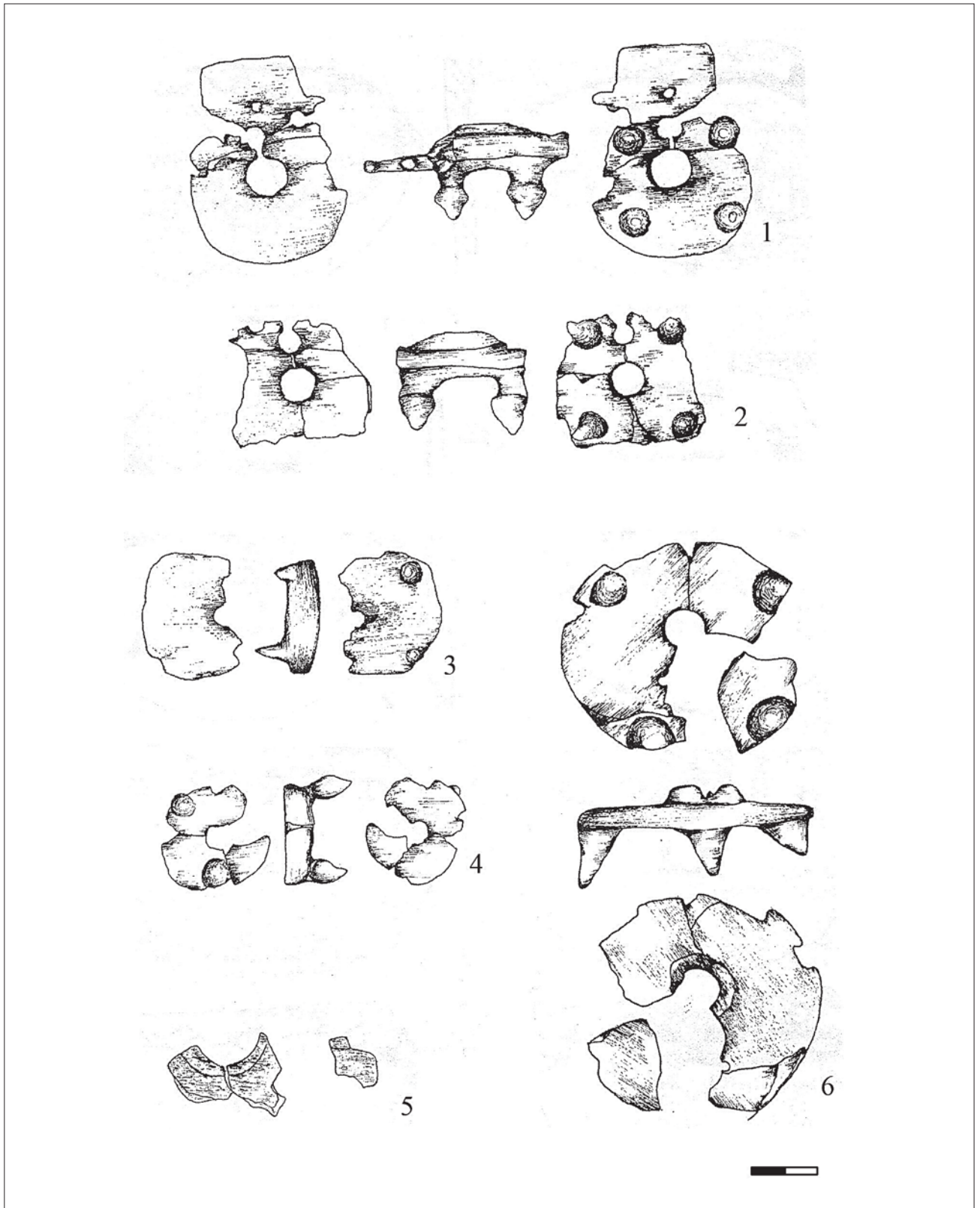
Рис. 30. Принадлежности конской упряжи из памятников синташтинского типа. Псалии 1-3 – могильник Танаберген II. Курган 7. Яма 22; 4 – могильник Танаберген II. Курган 7. Яма 23; 5-6 – могильник Танаберген II. Курган 7. Яма 33. По: (Ткачев, 2007)
