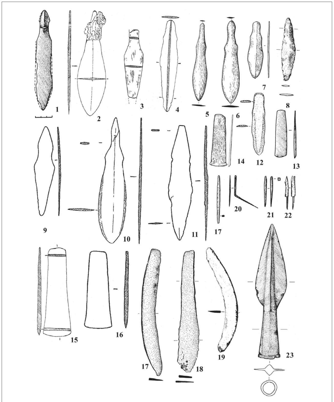
Рис. 51. Металлокомплекс памятников петровского типа. Орудия труда и предметы вооружения
