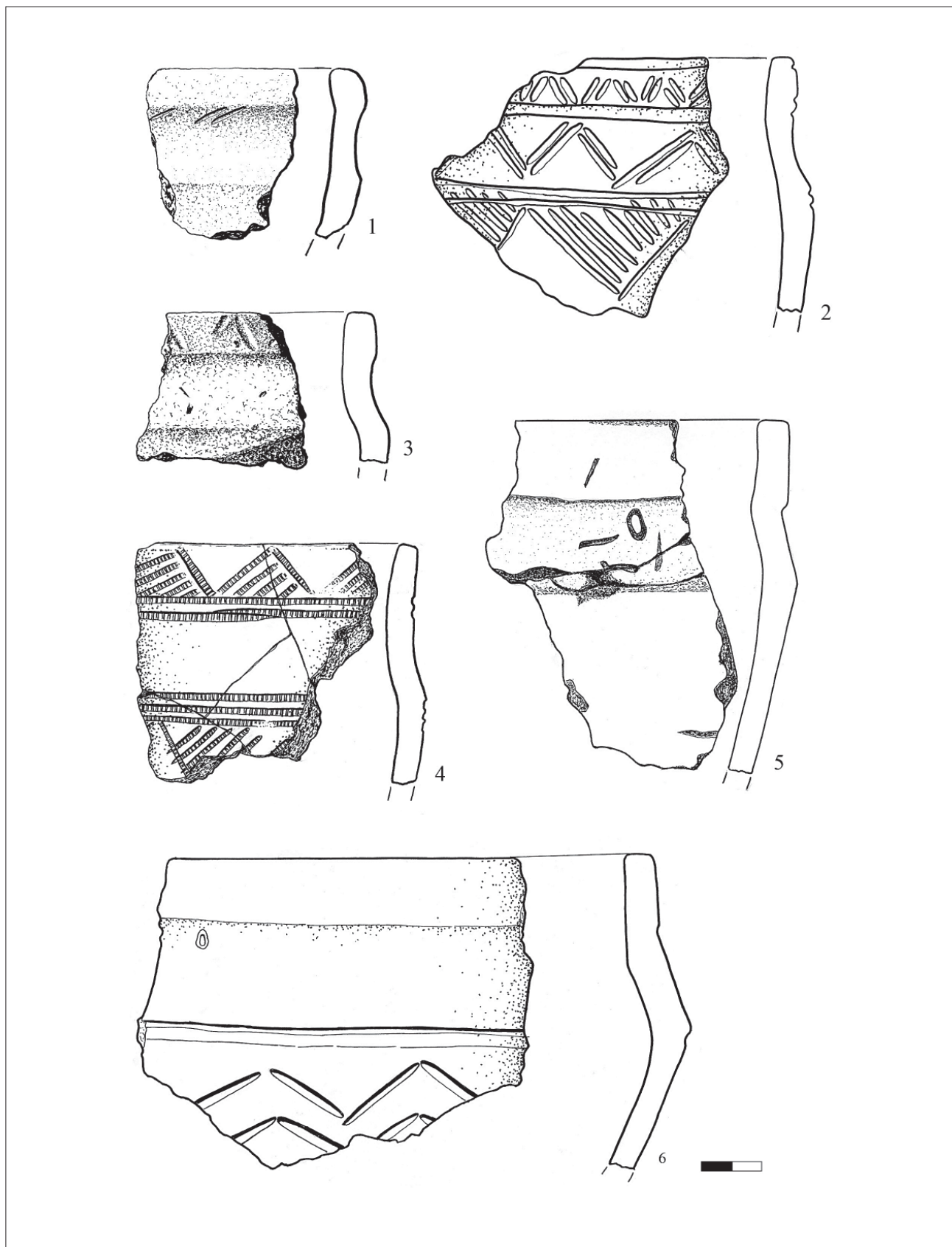
Рис. 44. Керамика памятников петровского типа 1-7 — укрепленное Устье I
