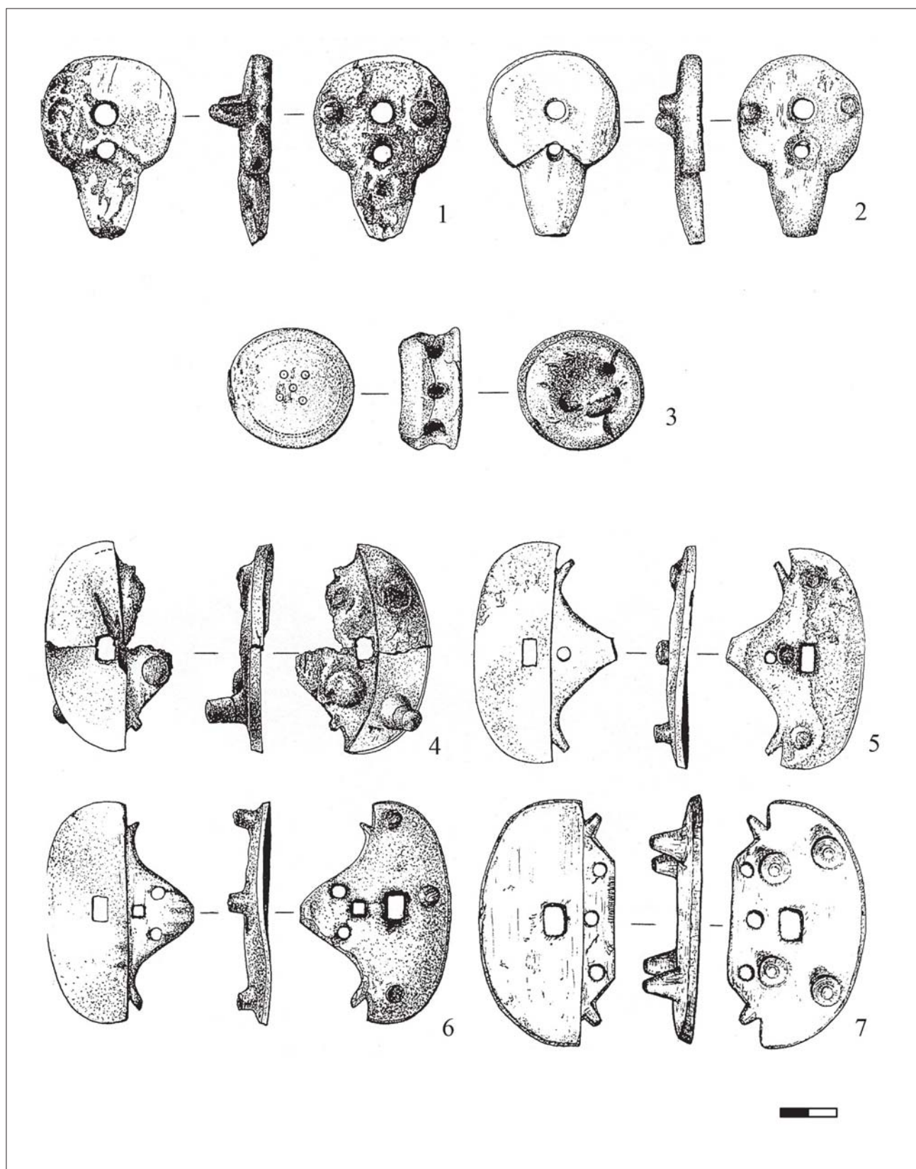
Рис. 53. Принадлежности конской упряжи из памятников петровского типа. Псалии 1, 2, 4-7 – псалии; 3 – распределитель ремней; 1-2 – могильник Кривое Озеро. Курган 1. Яма 3; 3-4 – могильник Кривое Озеро. Курган 1. Яма 2; 5-6 – могильник Кривое Озеро. Курган 1. Яма 1; 7 – могильник Кривое Озеро. Курган 2. Яма 1
