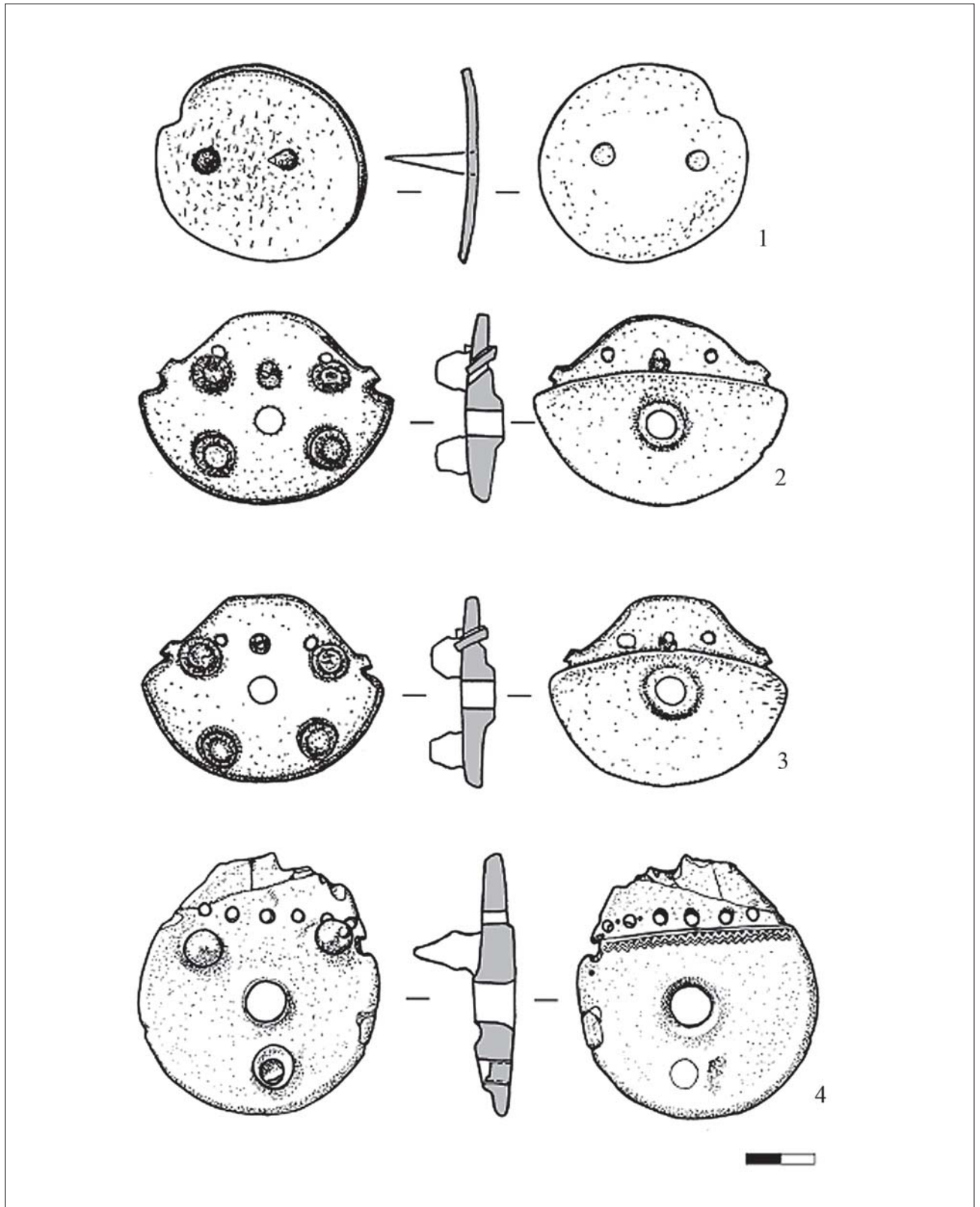
Рис. 28. Принадлежности конской упряжи из памятников синташтинского типа. Псалии 1-4 – могильник Каменный Амбар-5. Курган 2. Яма 8. По: (Епимахов, 2005)
