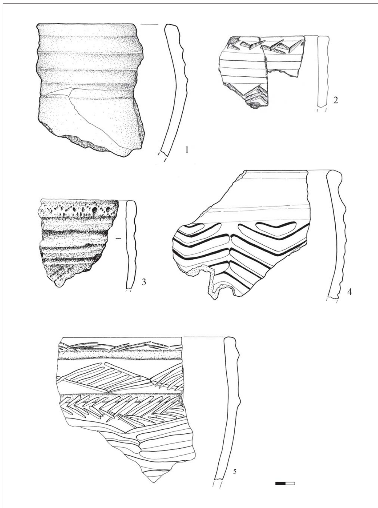
Рис. 5. Керамика памятников синташтинского типа 1-5 — укрепленное поселение Устье I
