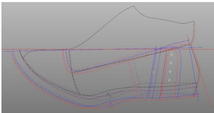
Рисунок 4. Чертеж деталей верха обуви
