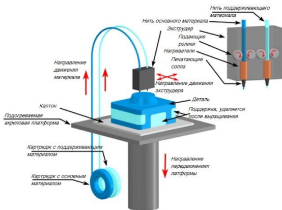
Рисунок 1 - Схема работы типичного FDM принтера
