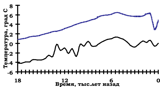
Рис. 2. Изменение температуры поверхности Земли за последние 18 тыс. лет [2, с. 145]. а – реконструированные по измерениям температуры в скважине Ильменская-1; б – полученные по исследованиям кернов льда в Гренландии
