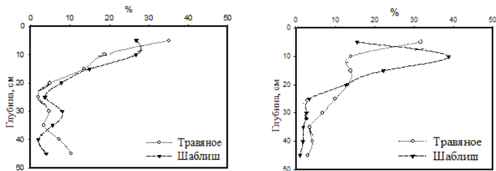
Рис. 2. Распределение (%) ^{90}\text{Sr} и ^{137}\text{Cs} в почвенных разрезах супераквальных ландшафтных элементов водосборов озер ВУРСа
