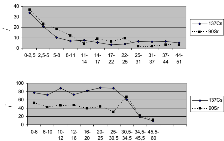
Рис. 2. Изменение удельной активности ^{90}\text{Sr} и ^{137}\text{Cs} по глубине почвенного профиля элювиальных позиций водосбора озер: а) Кожакуль; б) М. Кирпичики
