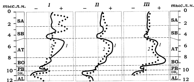
Рис. 3. Климатические колебания в голоцене
