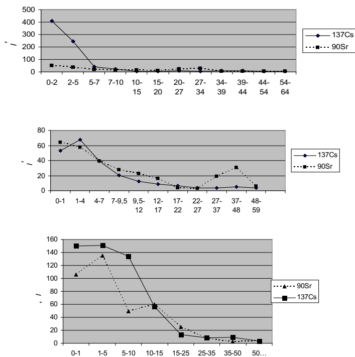
Рис. 1. Изменение удельной активности ^{90}\text{Sr} и ^{137}\text{Cs} по глубине профиля почв супераккумулятивных позиций водосбора озер: а) Кожакуль; б) М. Кирпичики; в) Куяш
