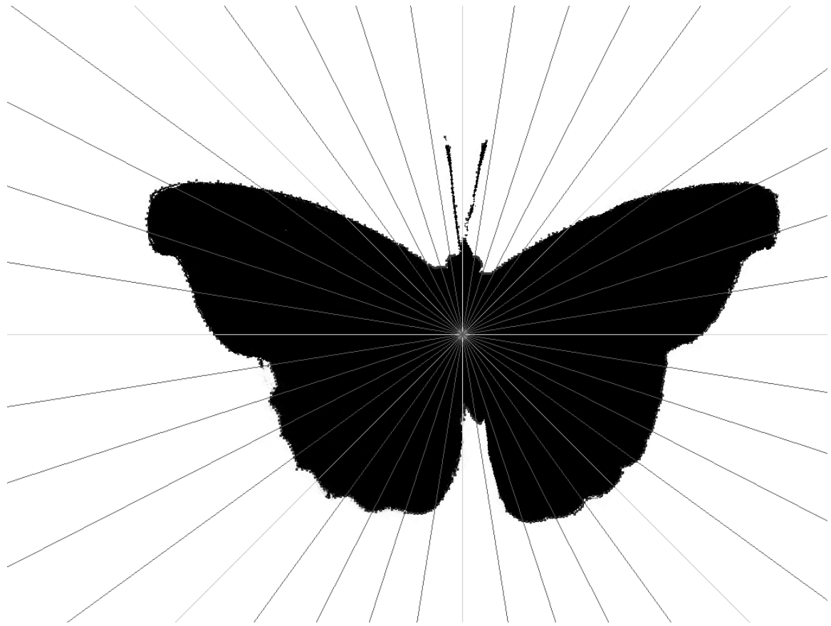
Рисунок 54 – Проекция бабочки в полярной системе координат, центр которой совмещен с геометрическим центром проекции
