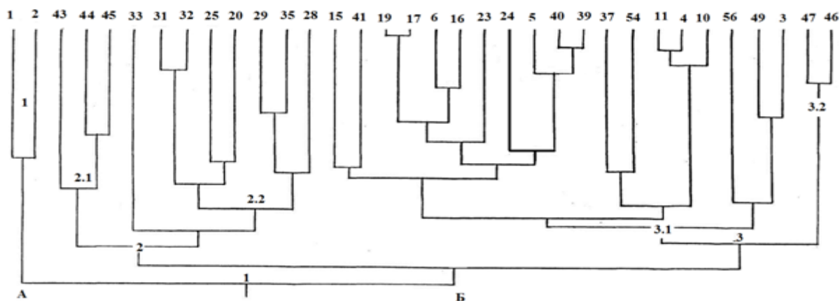
Рисунок 33 – Иерархия габитусов кокциnellид; А – тип габитуса « Epilachninae »; 1– форма габитуса «крупнотелые»; Б – тип габитуса « Coccinellinae »; 2 – форма габитуса «плоские»; 2.1 – вариант габитуса «узкотелые»; 2.2 – вариант габитуса «овальные»; 3 – форма габитуса «полусферообразные»; 3.1 – вариант габитуса «универсал»; 3.2 – вариант габитуса «шляпообразные» (номера объектов соответствуют номеру вида в таблице 2)
