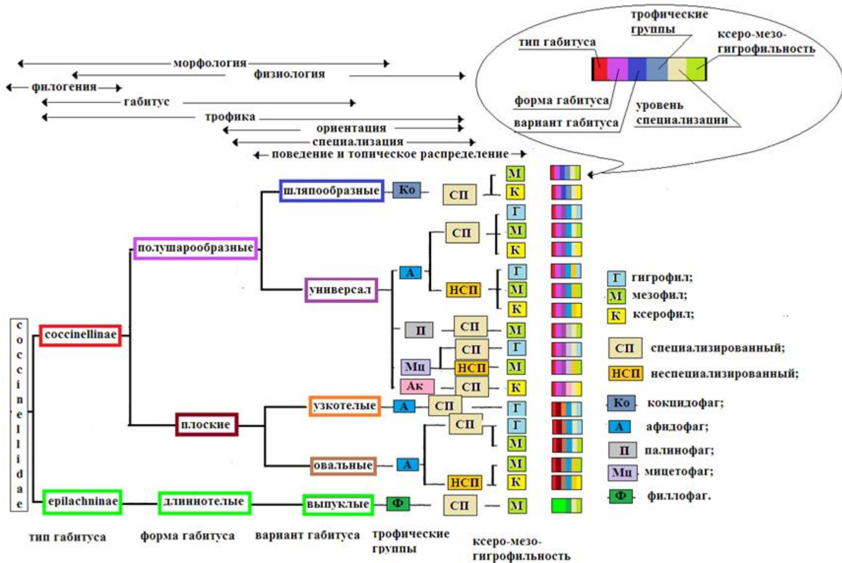
Рисунок 34 – Иерархическая система жизненных форм кокциnellид
