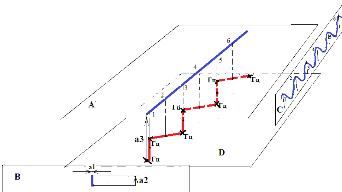
Рисунок 93 – Пространственная конфигурация локомоторной волны, генерируемой пенницей Aphrophora sp. при pedalной локомоции на пяти опорах; А, В, С – вид локомоторной волны в плоскости; D – плоскость опоры (крестиками обозначены геометрические центры площадей опор в различные моменты pedalной локомоции); a_1 – амплитуда движения центра тяжести тела в горизонтальной плоскости; a_2 – амплитуда движения центра тяжести тела в вертикальной плоскости; a_3 – расстояние от плоскости опоры до центра тяжести тела; красной линией показано смещение точки центра площадей опорных треугольников
