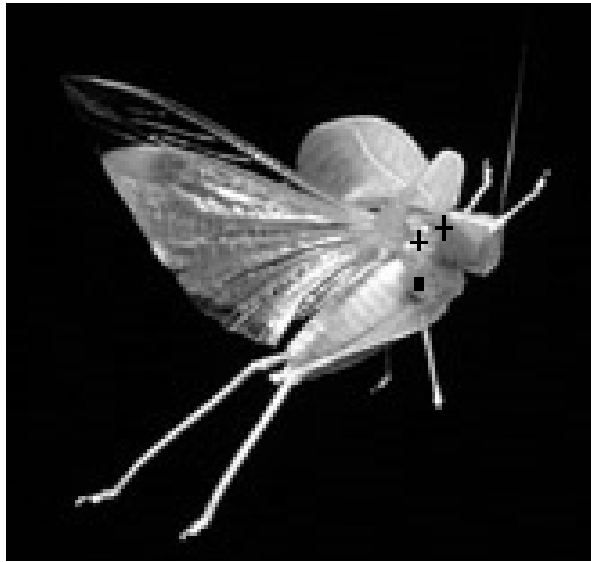
Рисунок 141 – Синфазный полет саранчовых и кузнечиков; Цт – центр тяжести тела; Цв з – центр вращения задних крыльев; Цв п – центр вращения передних крыльев
