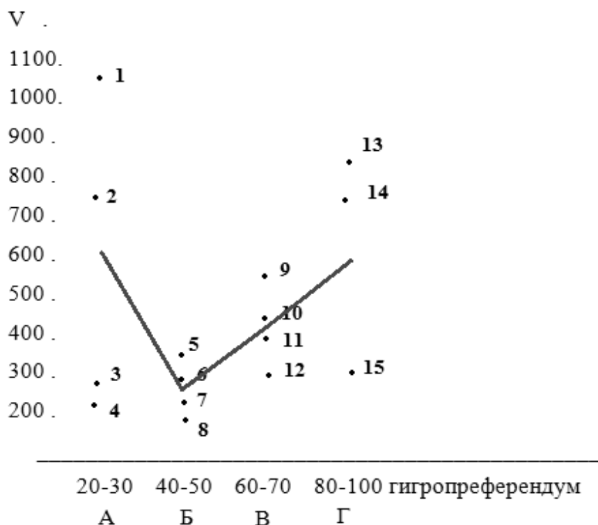
Рисунок 15 – Сравнение степеней неравномерности биотопического распределения (V) среди представителей различных экологических групп кокцинеллид: А – ксерофилы; Б – ксеро-мезофилы; В – гигро-мезофилы; Г – гигрофилы. 1 – Coccinula sinuatomarginata Fald; 2 – Hyperaspis reppensis Herbst.; 3 – Bulaea lichatschovi Hum.; 4 – Adonia variegata Goeze.; 5 – Tytthaspis lineola Gebl.; 6 – Propylaea 14-punctata L.; 7 – Coccinula 14-pustulata L.; 8 – Coccinella 7-punctata L.; 9 – Coccinella hieroglyphica L.; 10 – Synharmonia conglobata L.; 11 – Hippodamia 13-punctata L.; 12 – Thea 22-punctata L.; 13 – Pullus haemorrhoidalis Herbst.; 14 – Anisosticta 19-punctata L.; 15 – Coccidula rufa Herbst.
