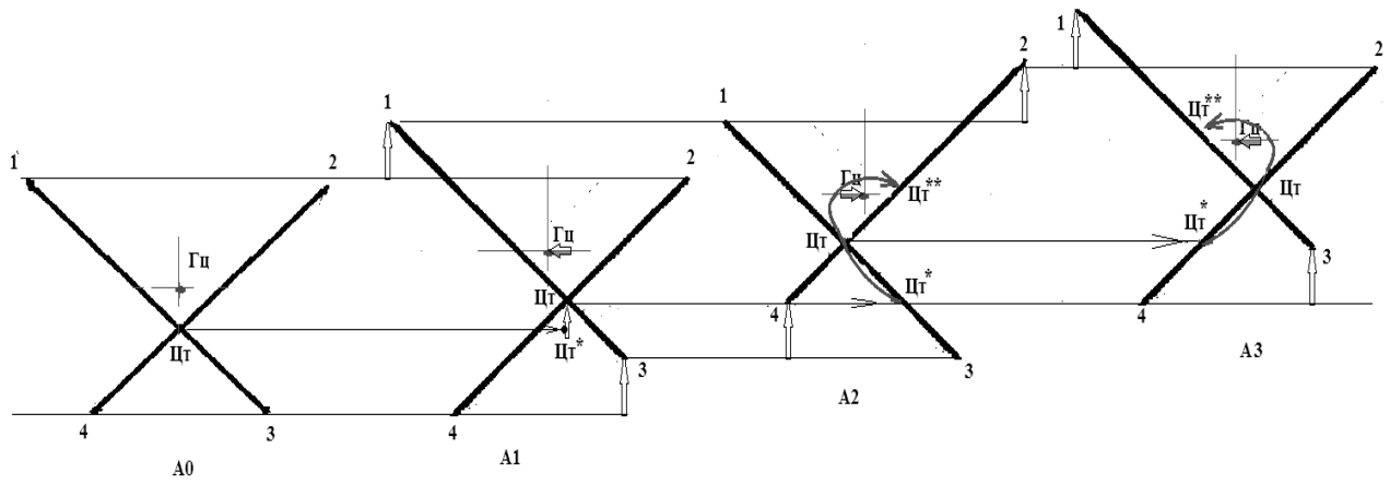
Рисунок 86 – Последовательность локомоторных актов Nymphalis antiopa L. при движении на четырех опорах (A0-A3); 1-4 – точки опоры; \Gamma_{ц} – геометрический центр площади опоры; \Pi_{г} – проекция центра тяжести на площадь опоры на момент локомоторного акта; \Pi_{г}^* – положение проекции \Pi_{г} на момент предыдущего локомоторного акта; \Pi_{г}^{**} – положение проекции \Pi_{г} на будущий локомоторный акт; стрелками показано смещение \Gamma_{ц} и \Pi_{г} в процессе локомоции
