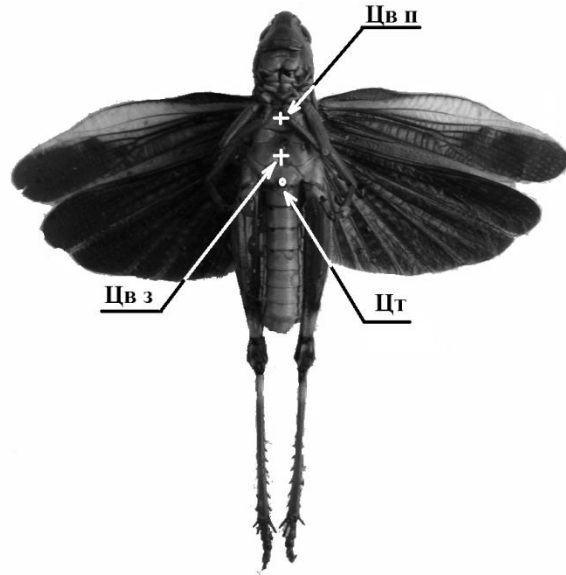
Рисунок 141 – Синфазный полет саранчовых и кузнечиков; Цт – центр тяжести тела; Цв з – центр вращения задних крыльев; Цв п – центр вращения передних крыльев
