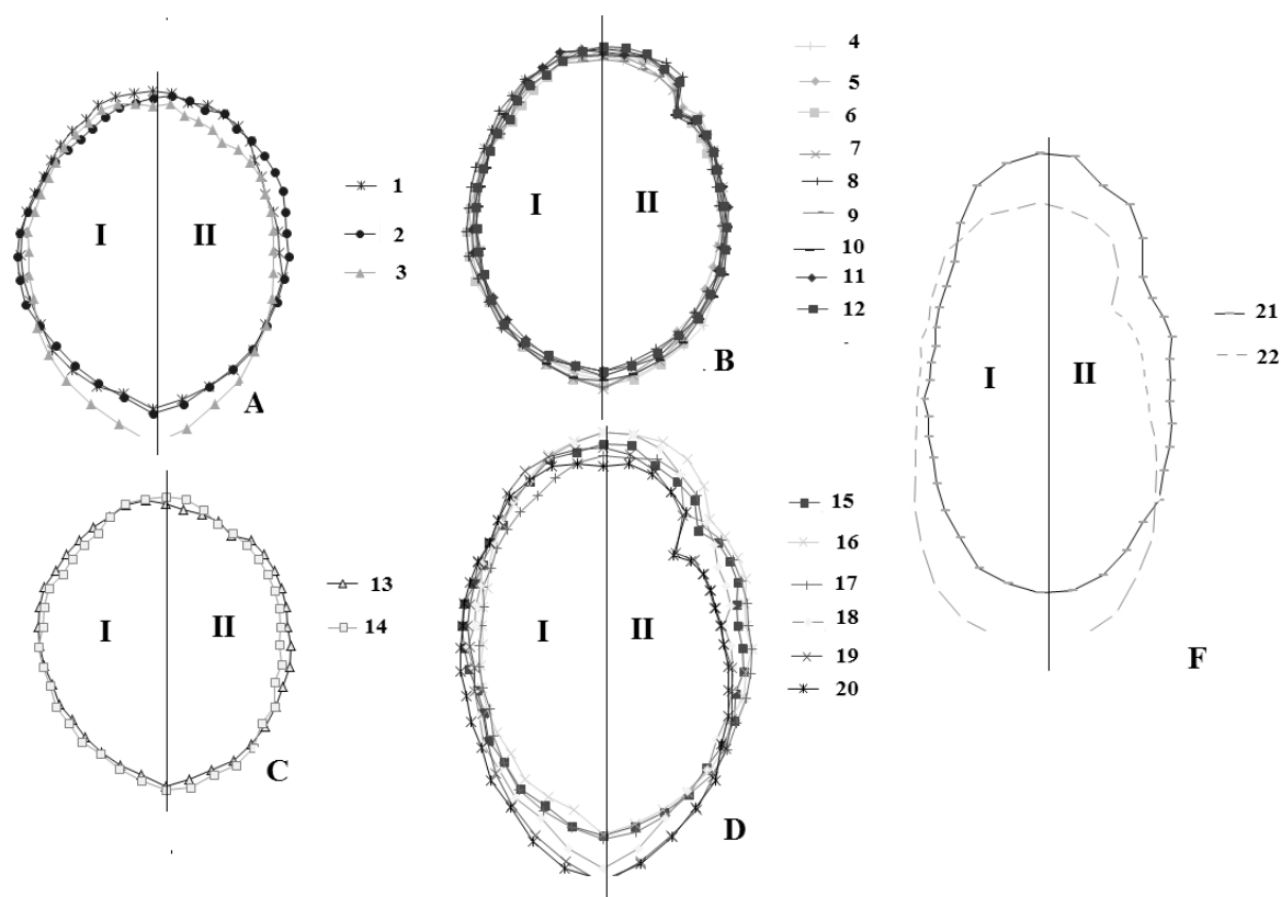
Рисунок 32 – Варианты габитуса кокциnellид: А – вариант «крупнотелые»; В – вариант «универсал»; С – вариант «шляпообразные»; Е – вариант «узкотелые»; D – вариант «овальные». I – латеральная проекция; II – правая сторона дорсовентральной проекции;
