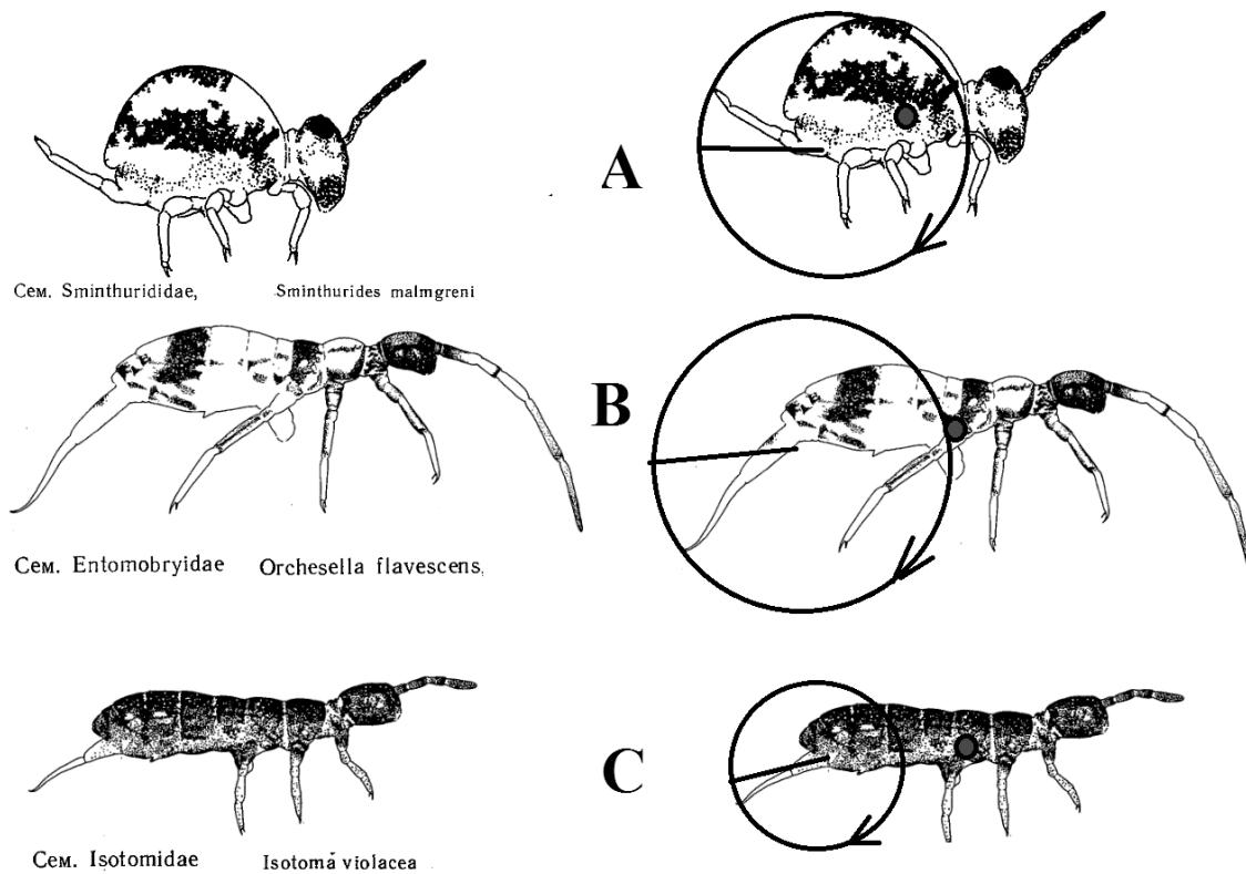
Рисунок 122 – Представители различных жизненных форм ногохвосток (по С.К. Стебаевой (1979) с изменениями); А – сминтуроидные поверхностные и верхнеподстилочные формы; В – энтомобриоидные атмобиотические формы; С – изотомоидные верхнеподстилочные формы; темным кружком обозначены центры тяжести тела; окружность радиусом, равным длине прыгательной вилки, описана относительно оси вращения прыгательной вилки; стрелки указывают направление вращения прыгательной вилки во время прыжка коллемболы
