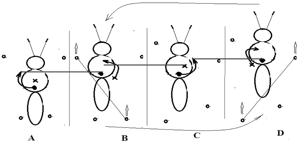
Рисунок 87 – Схема последовательности перемещения проекций центра тяжести ( \Pi_{г} ) тела Nymphalis antiopa L. (обозначены точкой) и геометрических центров ( \Gamma_{ц} ) площади опоры (обозначены крестиком) при локомоции на четырех опорах
