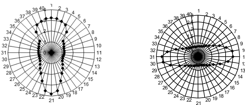
Рисунок 160 – Проекция нимфы и яйца Gryllus 2-maculatus Deg.
