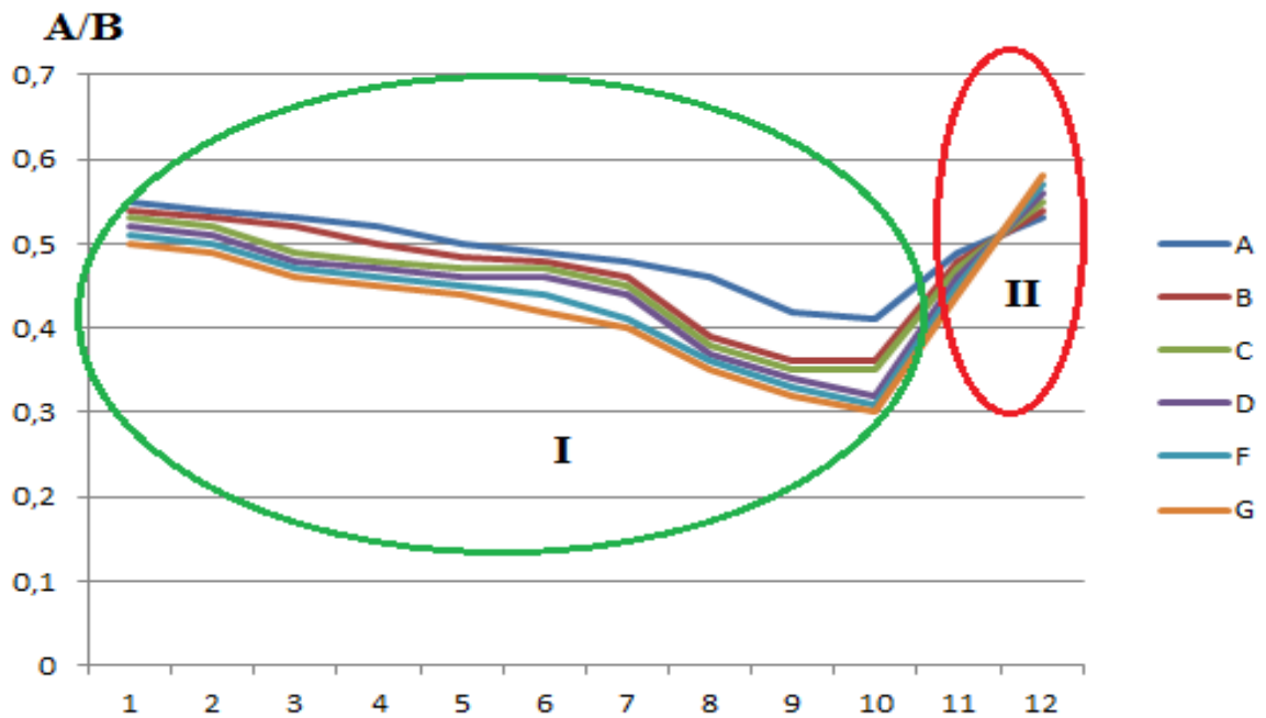
Рисунок 165 – Характер изменения величины A/B в периодах периодической системы жизненных форм имаго кокцинелл; A-G – периоды системы; I-II – группы; 1-10 – хищные кокцинеллы; II – группа 11 кокцинелл-мицетофагов и группа 12 кокцинелл-филлофагов
