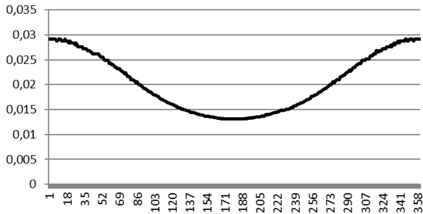
Рисунок 40 – Эквипотенциальная поверхность шара со смещенным центром тяжести в прямоугольной системе координат (по оси ординат – сопротивление качению ( 1/Rd ) в условных единицах, по оси абсцисс – поворот тела в градусах)
