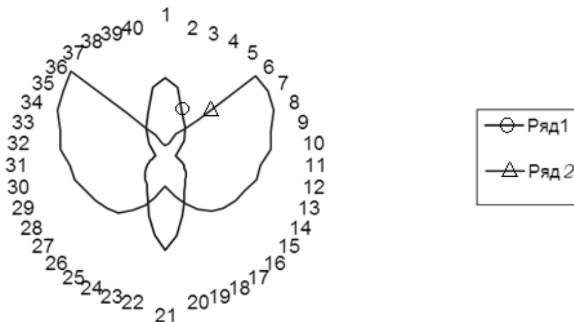
Рисунок 53 – Проекция тела бабочки (Ряд 1) и ее эквипотенциальная поверхность (Ряд 2); соотношение лучевых координат Ряда 1 (R1) и Ряда 2 (R2) описывается выражением: R1=1/R2 \cdot K ; где K – коэффициент пропорциональности
