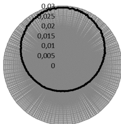
Рисунок 41 – Эквипотенциальная поверхность шара со смещенным центром тяжести в полярной системе координат, центр которой совмещен с центром тяжести шара (центр тяжести смещен в плоскости качения), по оси ординат – сопротивление качению ( 1/Rd )
