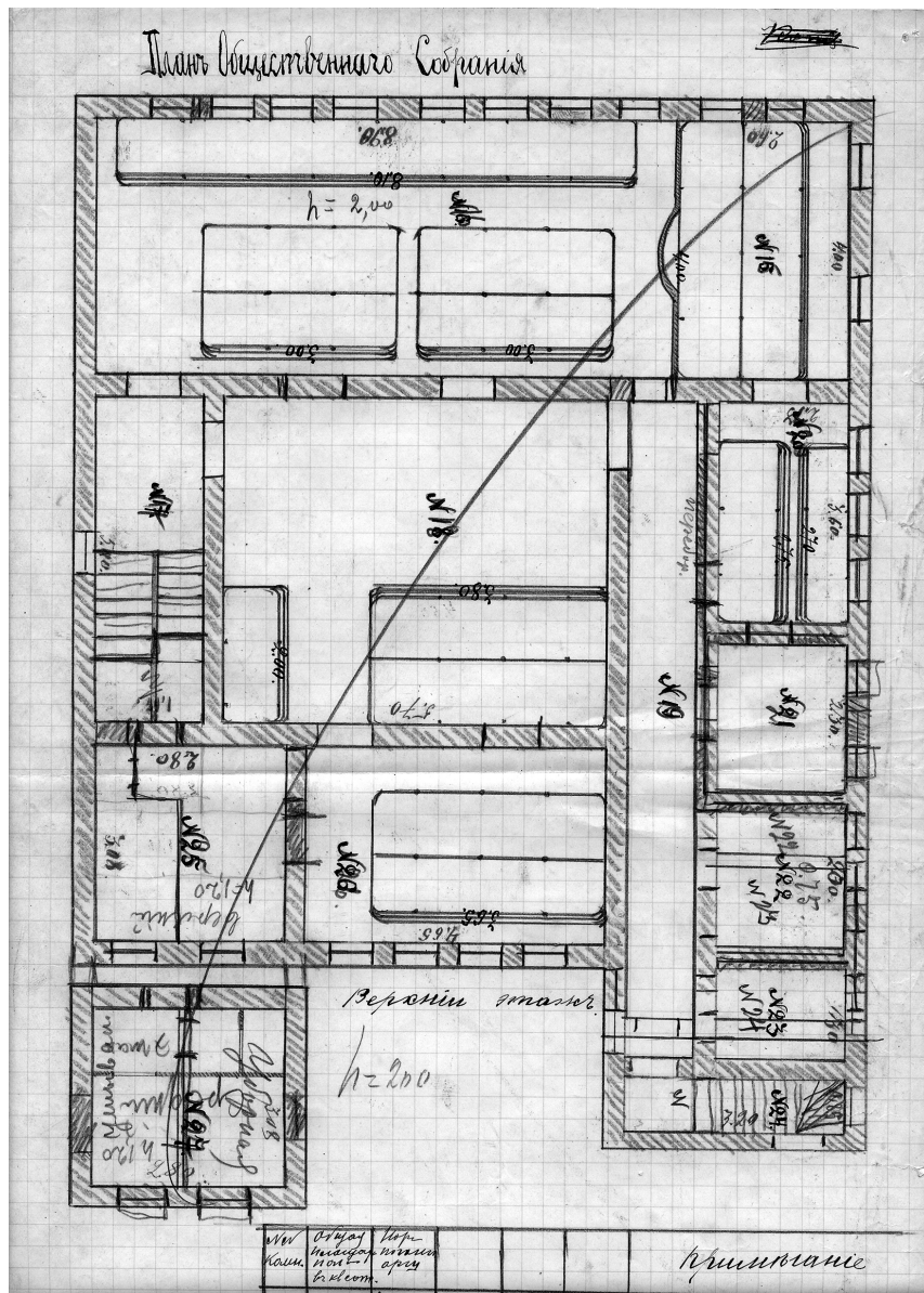
Илл. № 67. Челябинск. План дома общественного собрания
