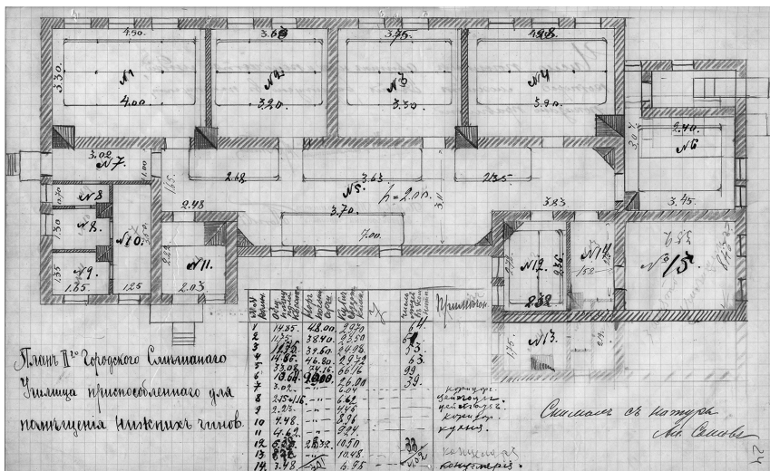
Илл. № 60. Челябинск. План II-го городского смешанного училища, приспособленного для помещения нижних чинов
